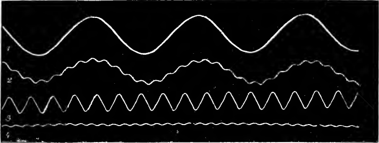
Fig. 22. — Tracés des vibrations de divers diapasons transmises par l'air. — Ligne 1, dix vibrations par seconde. — Ligne 2, 10 vibrations combinées à 80 par seconde. — Ligne 3, 50 vibrations par seconde. — Ligne 4, 100 vibrations par seconde. ( Héliogravure. )
